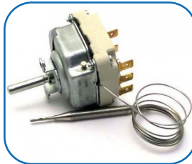
Ego-Capillary-Thermostat- 400v-16a-tmin-50a-c-tmax- 300a-c-88 FOR FRYER
